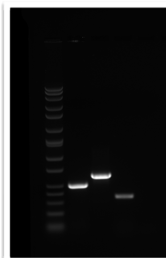
Gel de agarosa en la que se identifican de izquierda a derecha 3 genes de resistencia a macrólidos (mefA, ermB y ermTR) en Streptococcus pyogenes .
